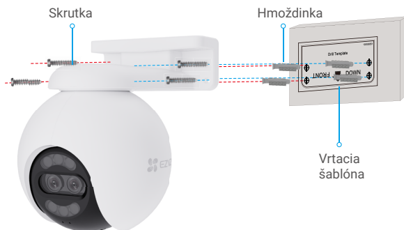
Fig. 2 Montáž na stenu
